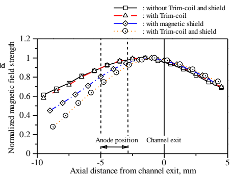
図3 磁場強度分布
